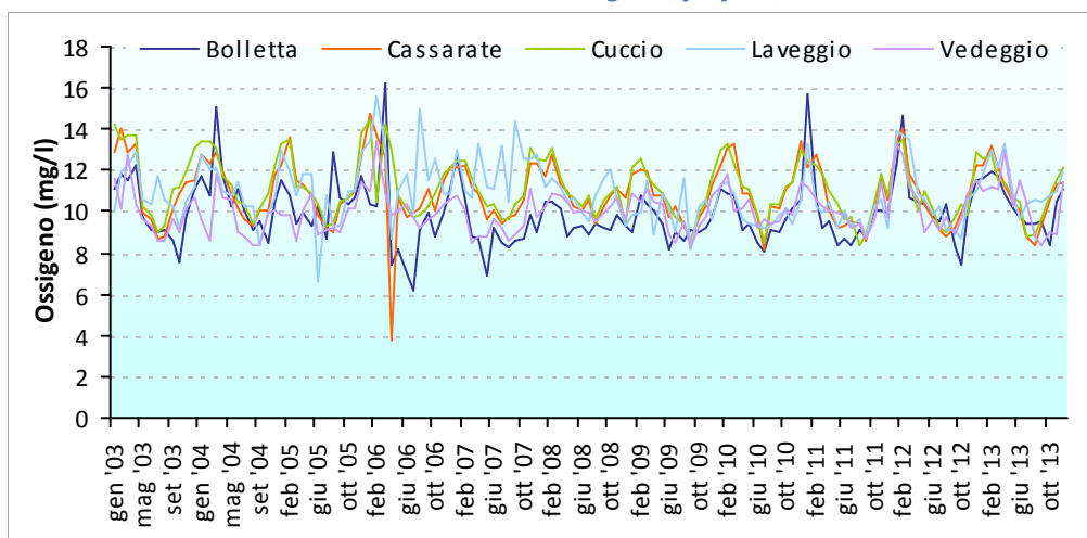
Andamento dei valori mensili di ossigeno, fosforo, azoto ammoniacale e azoto nitrico nei principali tributari del Lago di Lugano durante il periodo 2003-2013
