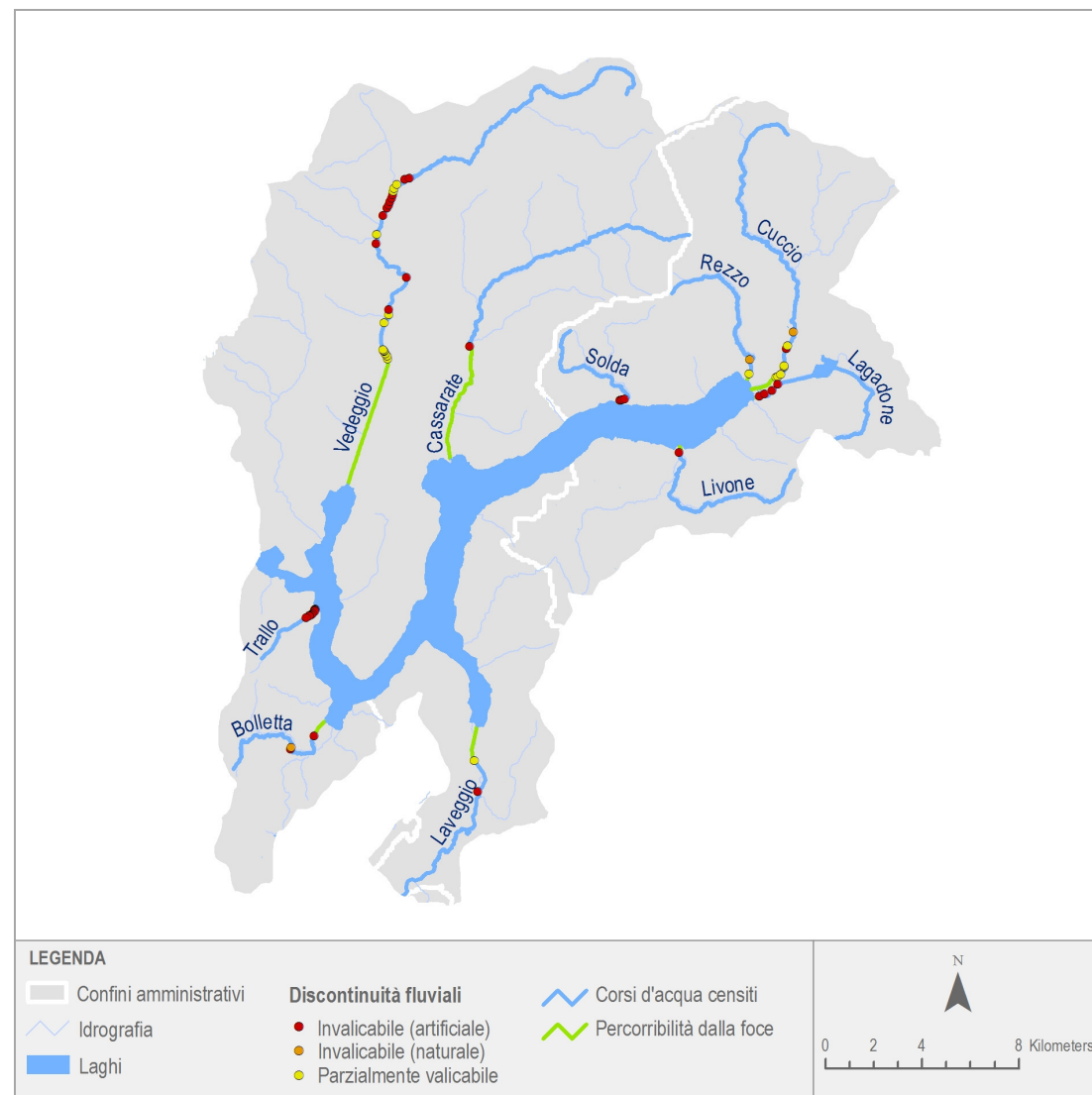
Carta delle discontinuità e della percorribilità fluviale nei principali immissari del Lago di Lugano La condizione delle percorribilità al 2013 conferma quanto rilevato nel 2010
