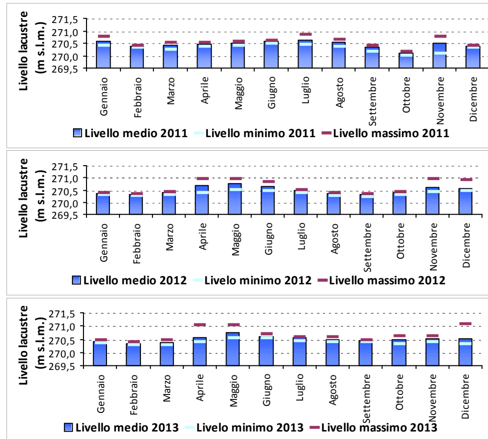
Livello lacustre* negli anni 2011, 2012, 2013: valori minimo, medio, massimo mensili
