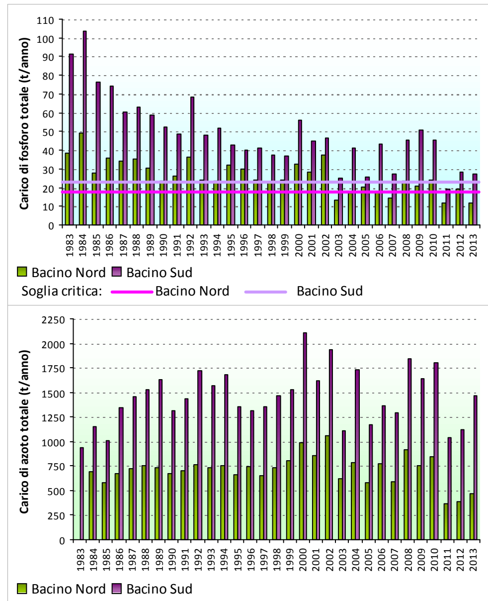
Apporti di nutrienti a lago, dal 1983 al 2013: fosforo totale (in alto) e azoto totale (in basso)
