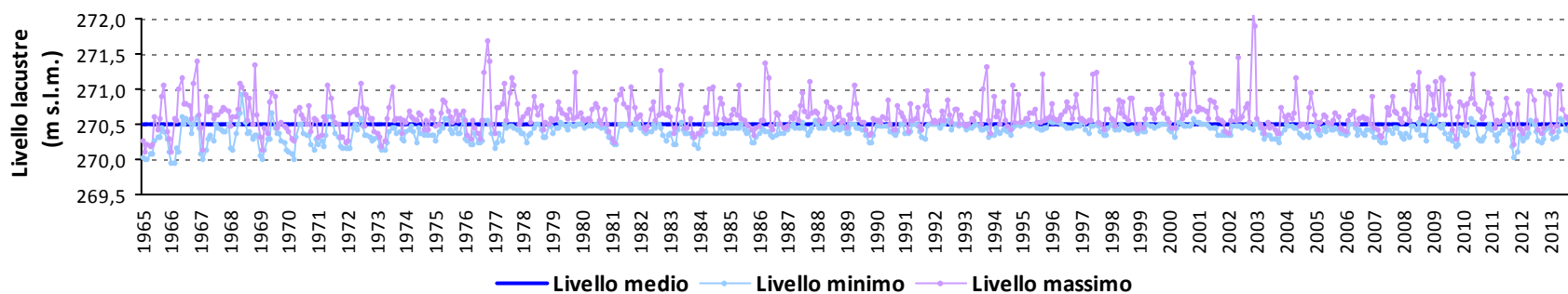
Andamento dei livelli lacustri minimi e massimi mensili* lungo la serie storica raffrontati con il livello medio lacustre di riferimento
