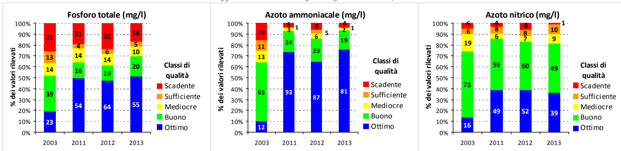
Ripartizione in classi di qualità dei valori mensili di fosforo totale, azoto ammoniacale e azoto nitrico rilevati nelle stazioni di monitoraggio dei tributari del Lago di Lugano: anni 2011, 2012 e 2013
