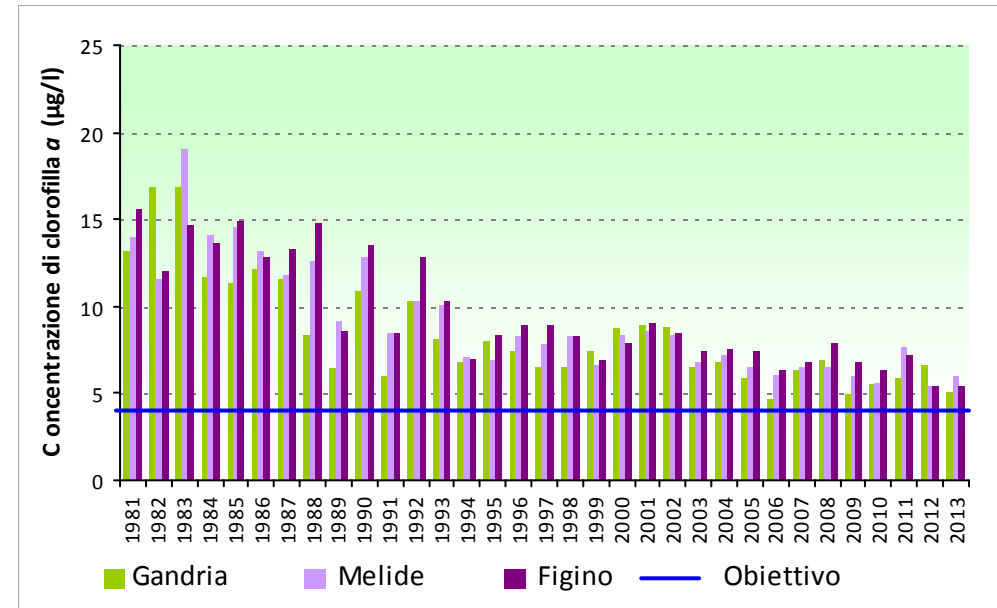
Concentrazione di clorofilla a: serie storica del valore medio annuo (in alto) e valori medi mensili per gli anni 2011, 2012, 2013 (in basso)
