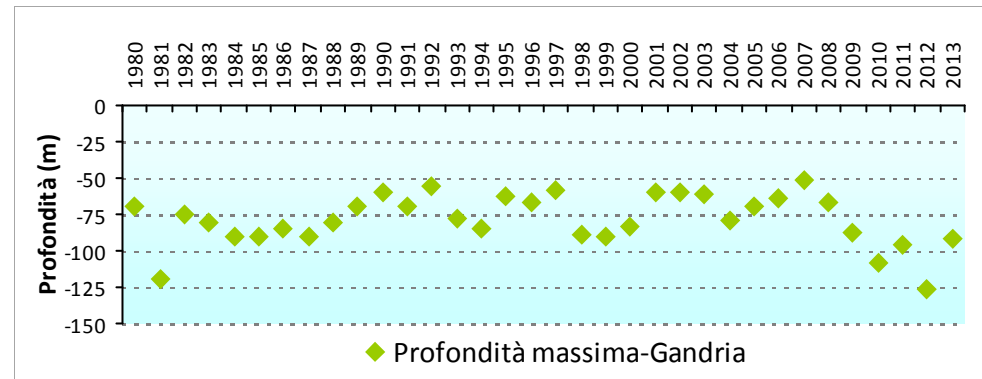
Profondità massima del Lago di Lugano a cui è stata rilevata una concentrazione di ossigeno pari a 4 mg/l nelle acque
